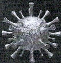
A/H1N1
